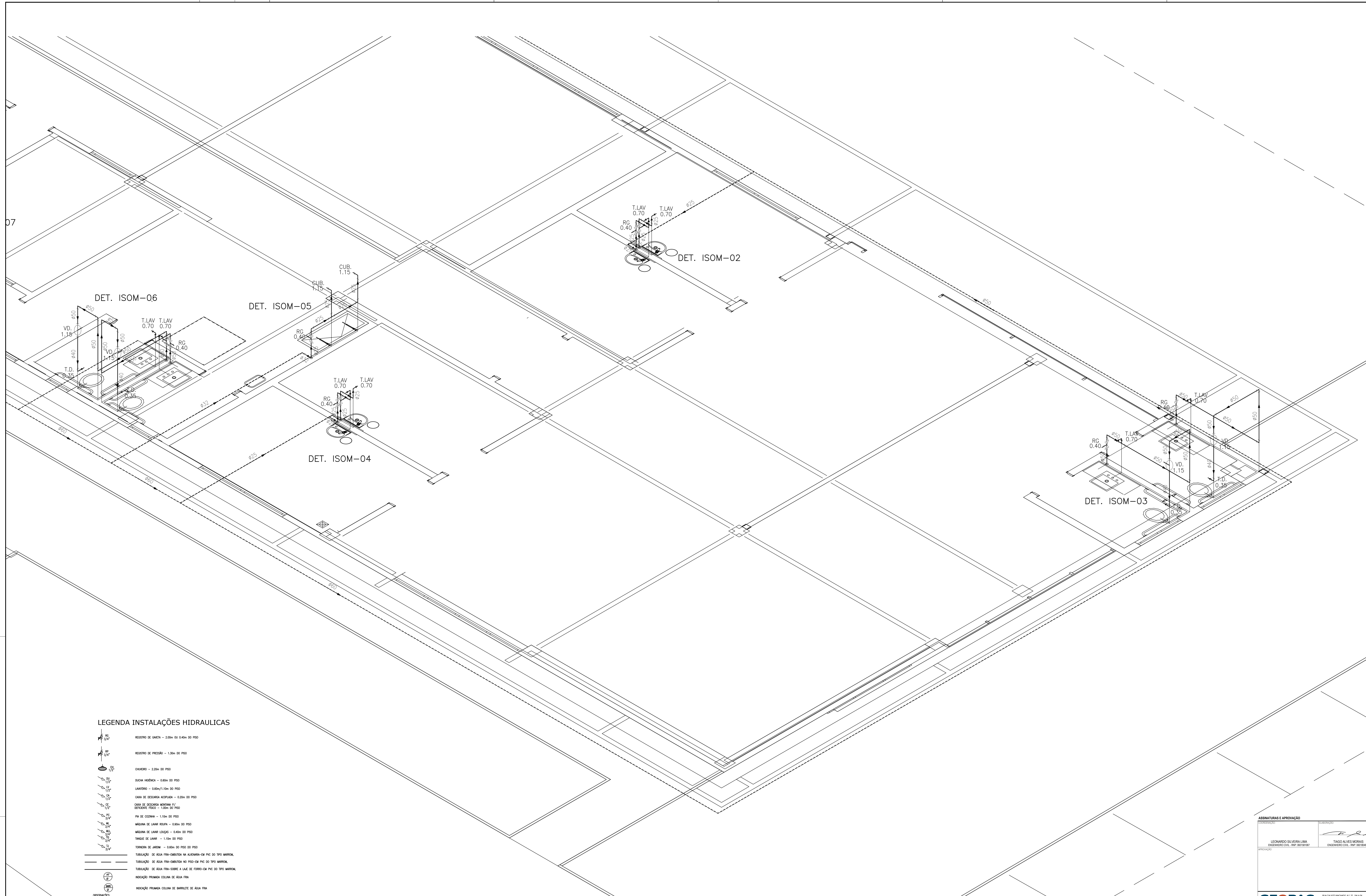
① DETALHE ISOMÉTRICO-TRECHO 2 1:50
